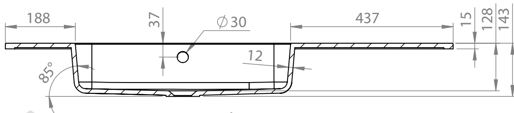
PRZEKRÓJ N-N SKALA 1 : 10
